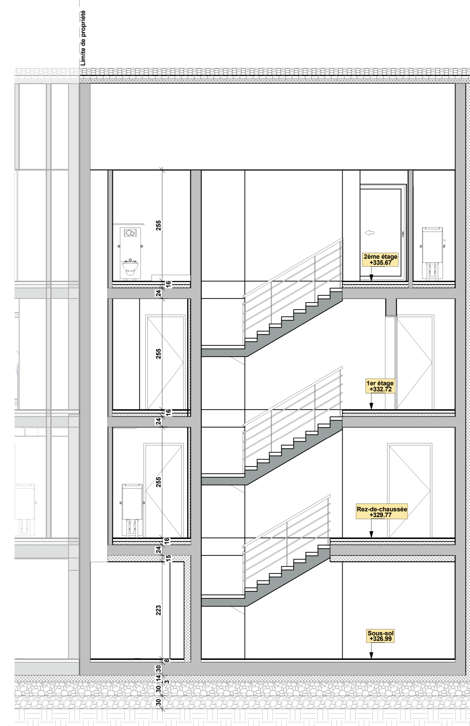
4 C6. Coupe B-B Ech. : 1 : 50
