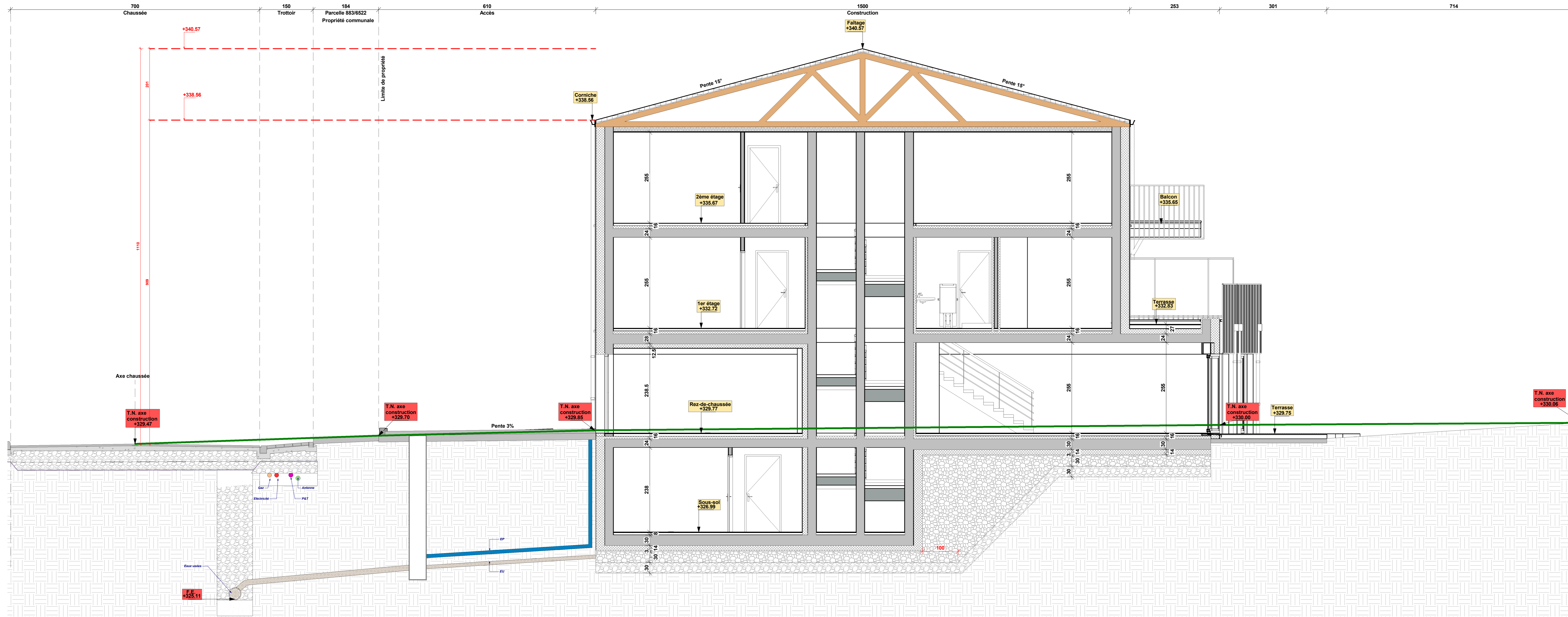
1 C5. Coupe A-A Ech. : 1 : 50
